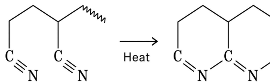
< 화학구조 변화 >
