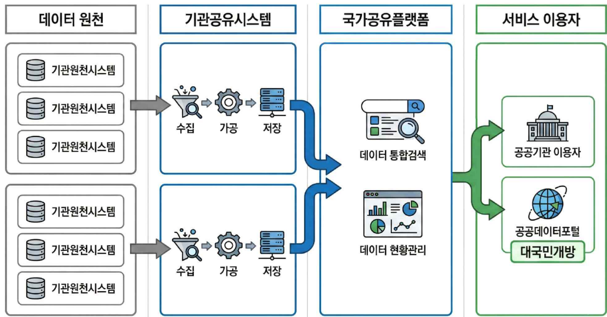
< 범정부 데이터 파이프라인 구성도 >
