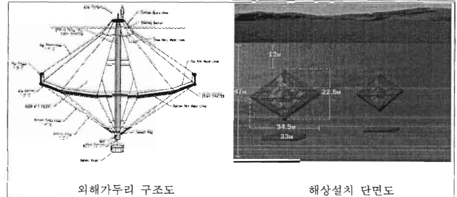
외해가두리 구조도
